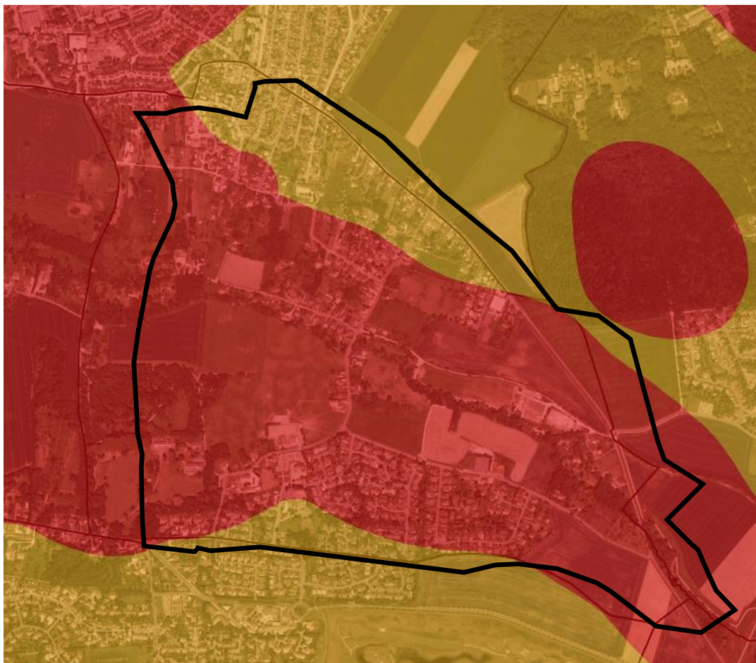
Carte d'exposition au retrait-gonflement des argiles - Source : Géorisques - BRGM
