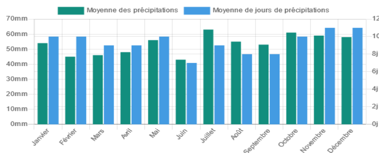
Météo à Conches-sur-Gondoire (Source : Météo France, 2021)
