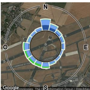
Distribution de la direction du vent (Station de Paris-Le Bourget, moyenne annuelle; Source : windfinder.com)
