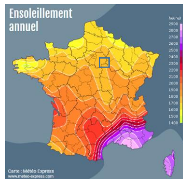
Carte de l'ensoleillement (Source : météoexpress.fr)
